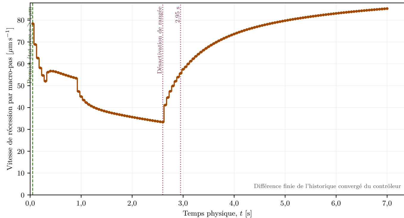
Vitesse de récession du secteur fin en fonction du temps
