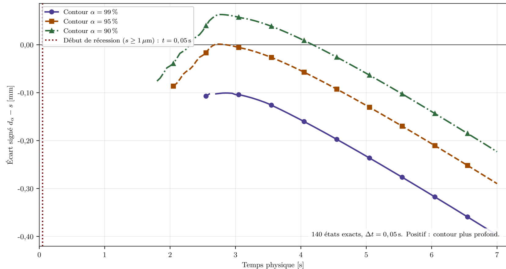
Simulation 3 : écart radial entre la récession virtuelle et les contours de conversion pyrolytique
