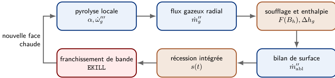
Figure 5. Chaîne physique proposée pour la simulation 2 dans Mechanical. La suppression est pilotée par la récession, non directement par SVAR1.
