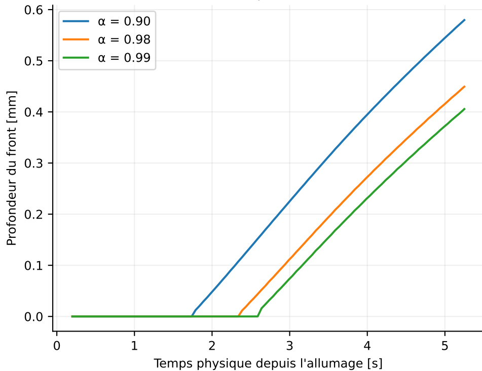
Front continu depuis la face chaude
