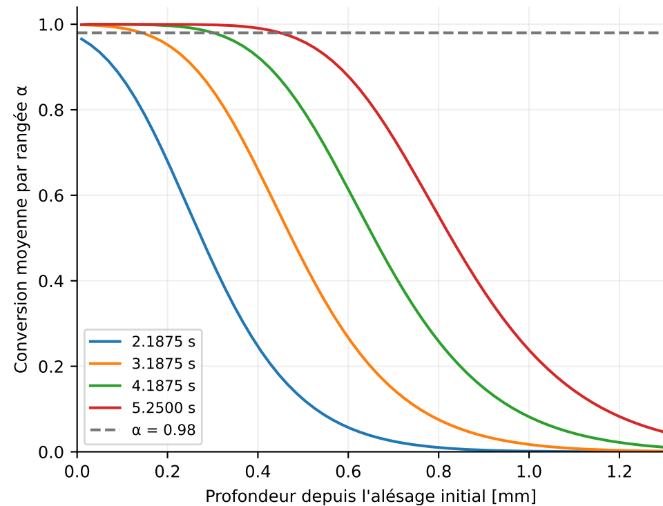
Profils radiaux de conversion
