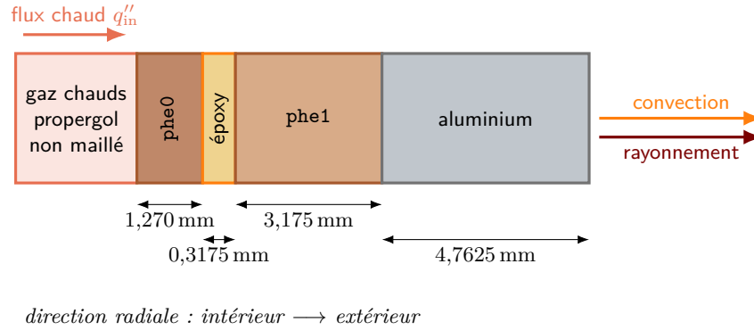
Figure 1. Empilement radial nominal corrigé. La largeur des couches est schématique ; les cotes indiquées sont les épaisseurs radiales.
