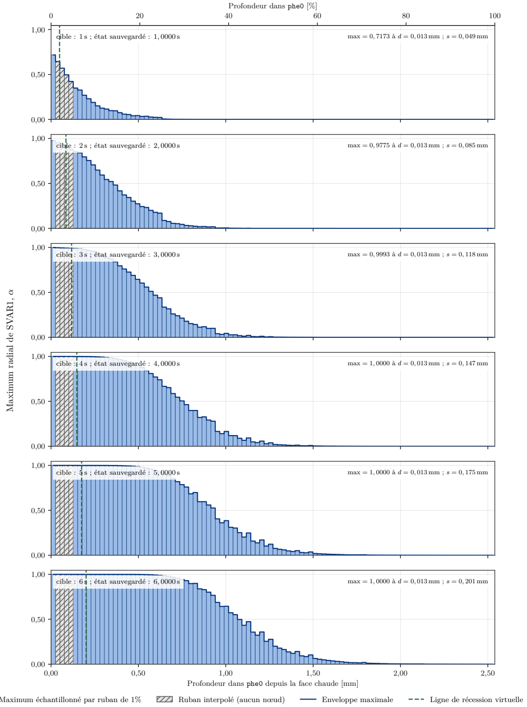
Figure 14. Évolution du maximum radial de SVAR1 dans la simulation 2. La ligne verte discontinue indique, dans chaque panneau, la position cumulée de la récession virtuelle.
