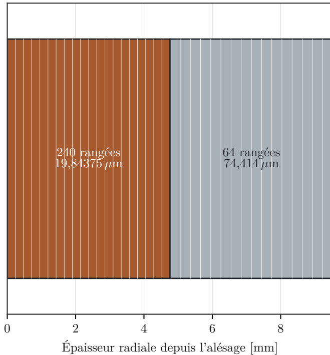
Discrétisation radiale
