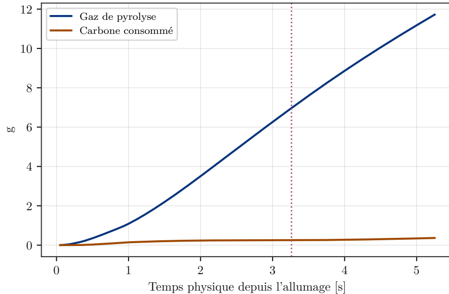
Masses cumulées : anneau complet, L = 50 \text{ mm}
