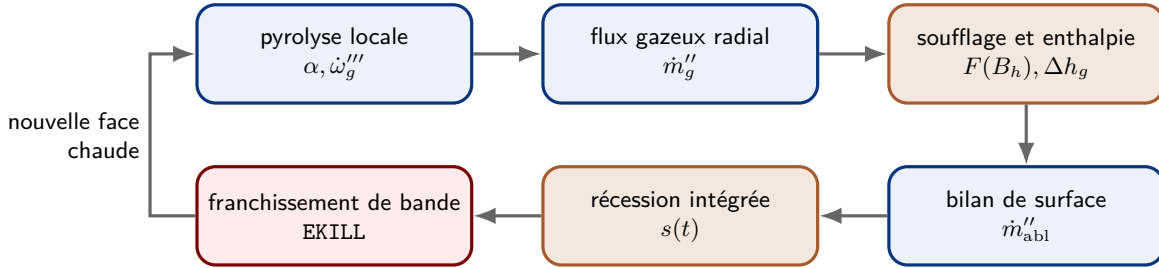
Figure 3. Chaîne physique proposée pour la simulation 2 dans Mechanical. La suppression est pilotée par la récession, non directement par SVAR1.
