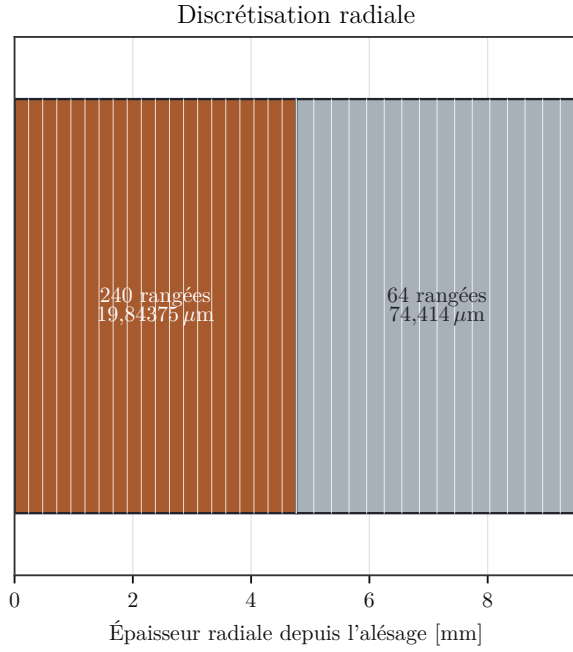
Figure 2. Résolution radiale et inventaire du maillage final.
