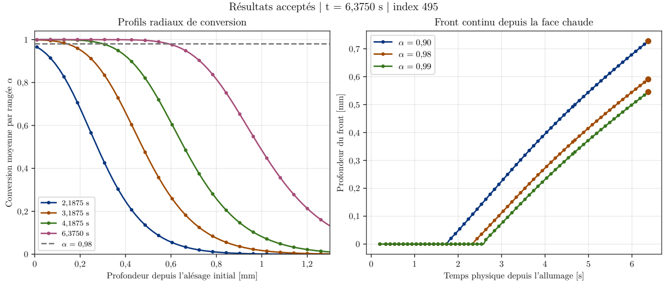
Figure 4. Profils de conversion et profondeurs des fronts à 90, 98 et 99 %. Les profils montrent les premiers 1,3 mm des 4,7625 mm initiaux. Les historiques des fronts utilisent un checkpoint sur quatre, complété par le dernier état accepté et le checkpoint de comparaison précédent.
