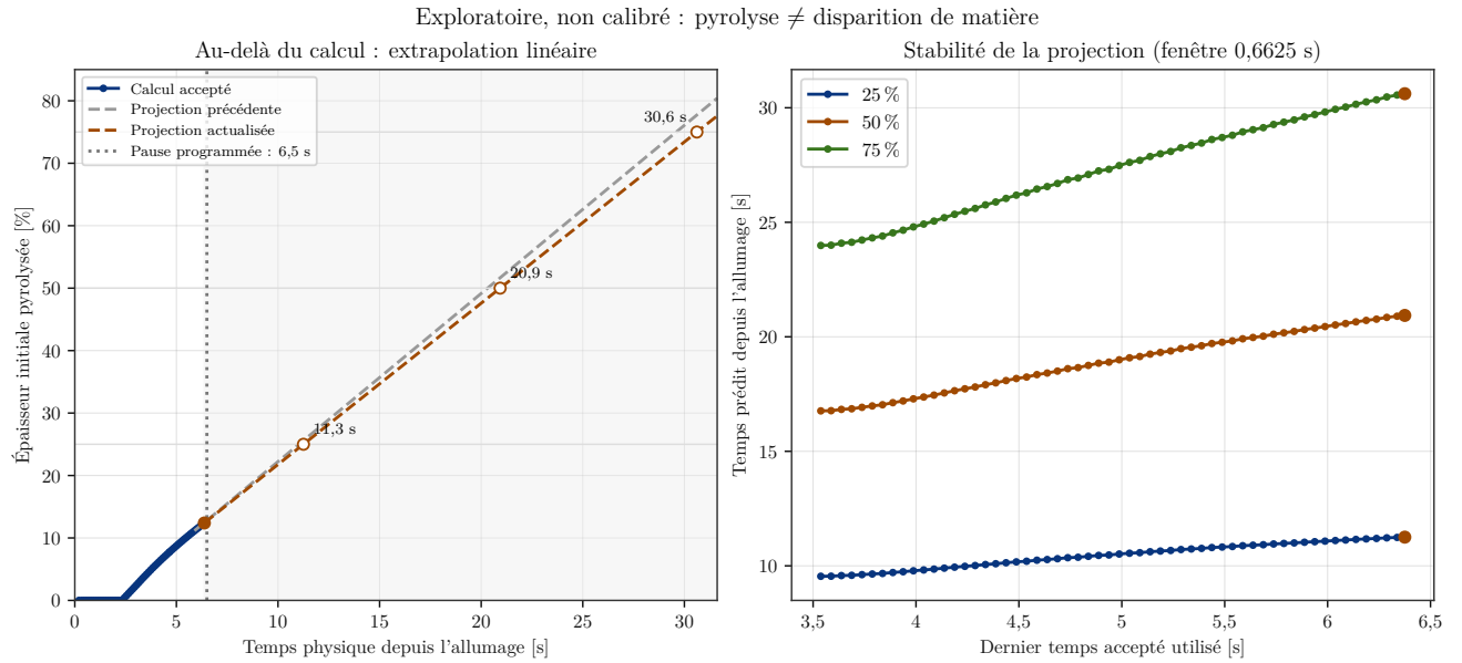
Figure 5. À gauche, calcul accepté en trait plein et extrapolations en tirets ; la zone grise est au-delà des résultats disponibles. À droite, dérive des temps prédits lorsque de nouveaux checkpoints entrent dans la fenêtre d'ajustement.
