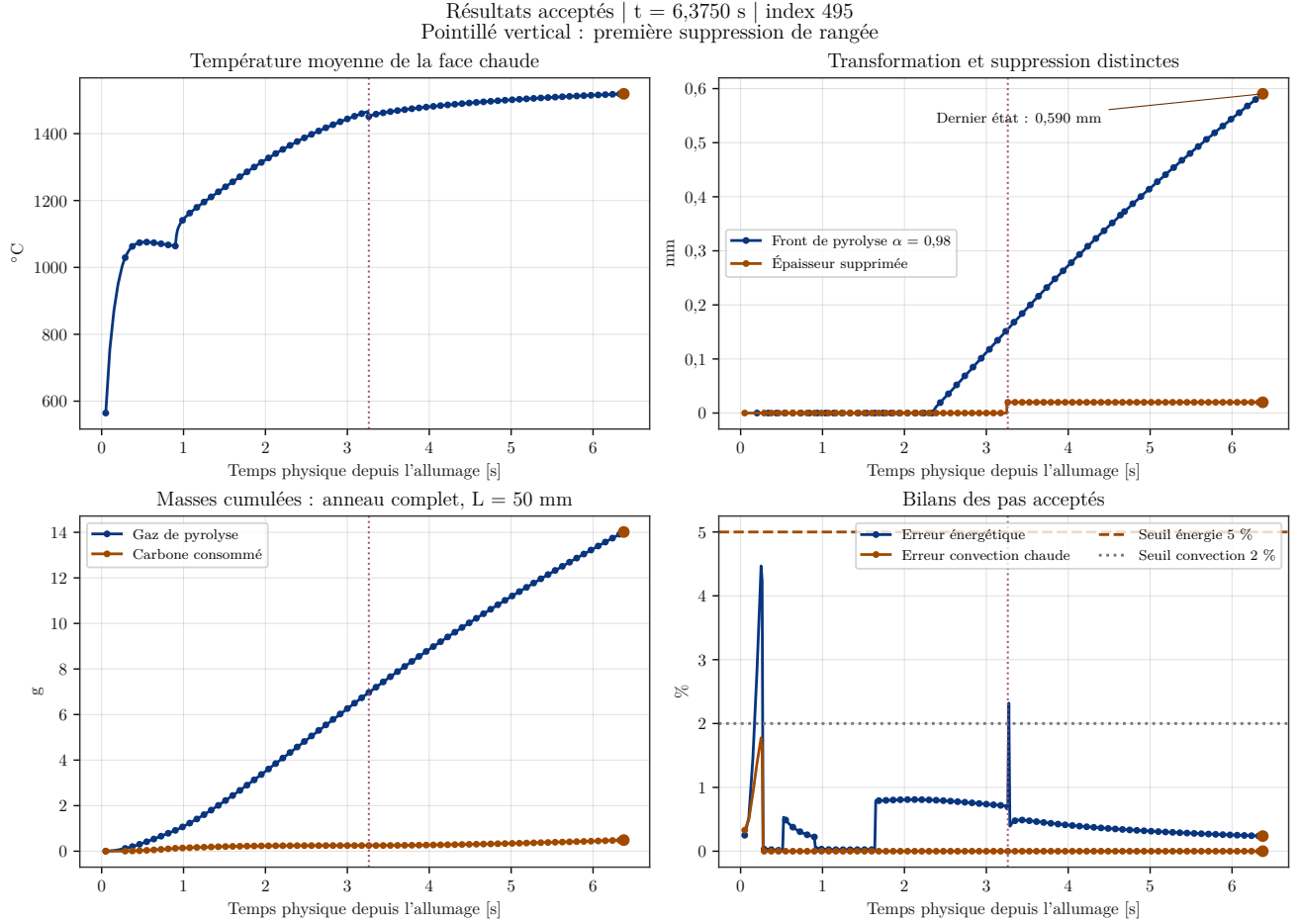
Figure 3. Historique accepté : température moyenne de face chaude, profondeur pyrolysée et suppression géométrique, masses cumulées et erreurs de bilans. Les masses sont ramenées à un anneau complet de longueur 50 mm. Le pointillé vertical indique la première suppression de rangée.
