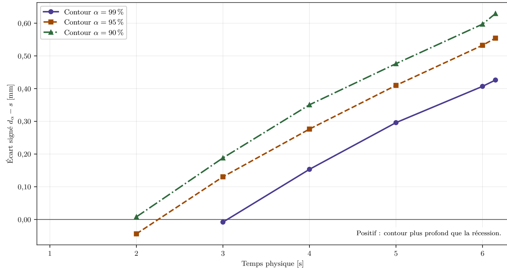
Simulation 2 : écart radial entre la récession virtuelle et les contours de conversion pyrolytique
