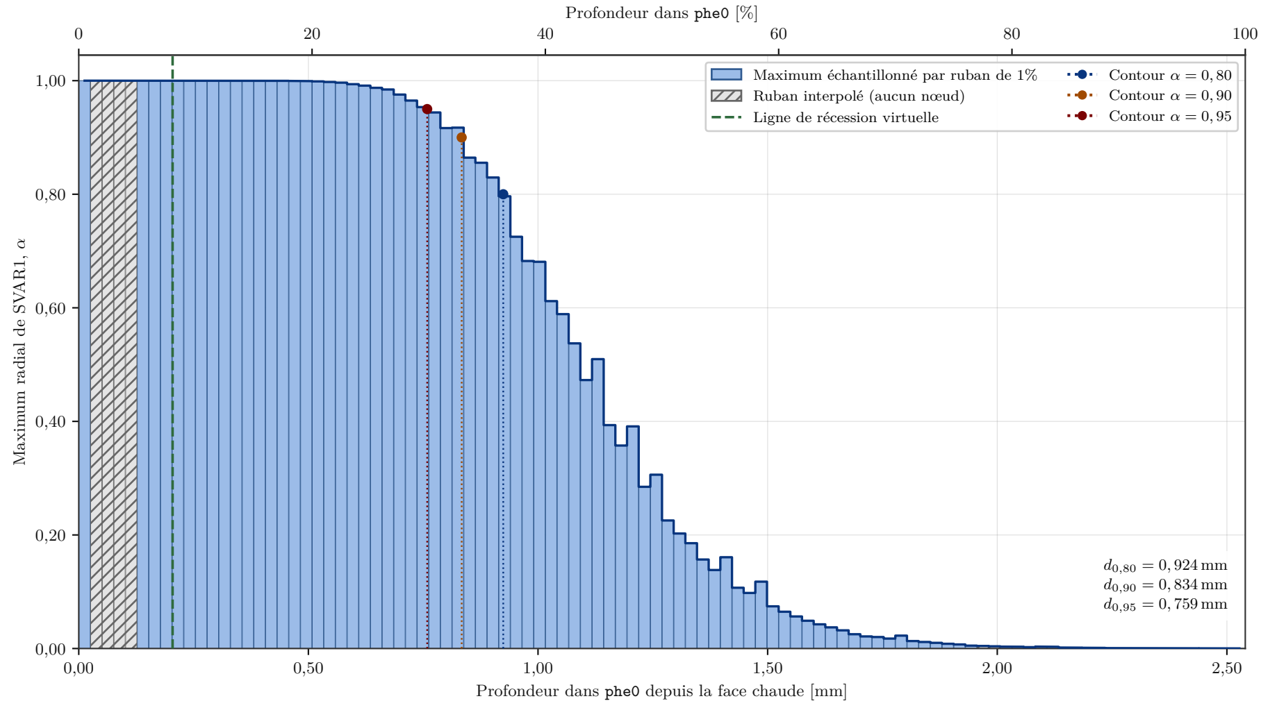
Simulation 2 : profil radial de SVAR1 au dernier état extrait t = 6,1500 \text{ s} ; ligne de récession s = 0,204 \text{ mm}
