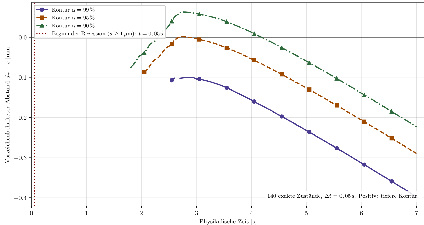
Simulation 3: radialer Abstand zwischen virtueller Rezession und Pyrolyse-Umsatzkonturen
