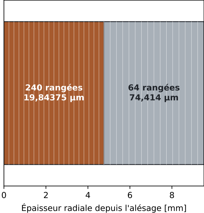
Discrétisation radiale
