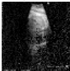
SegFormer
