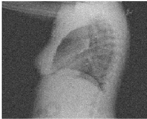
Noisy
