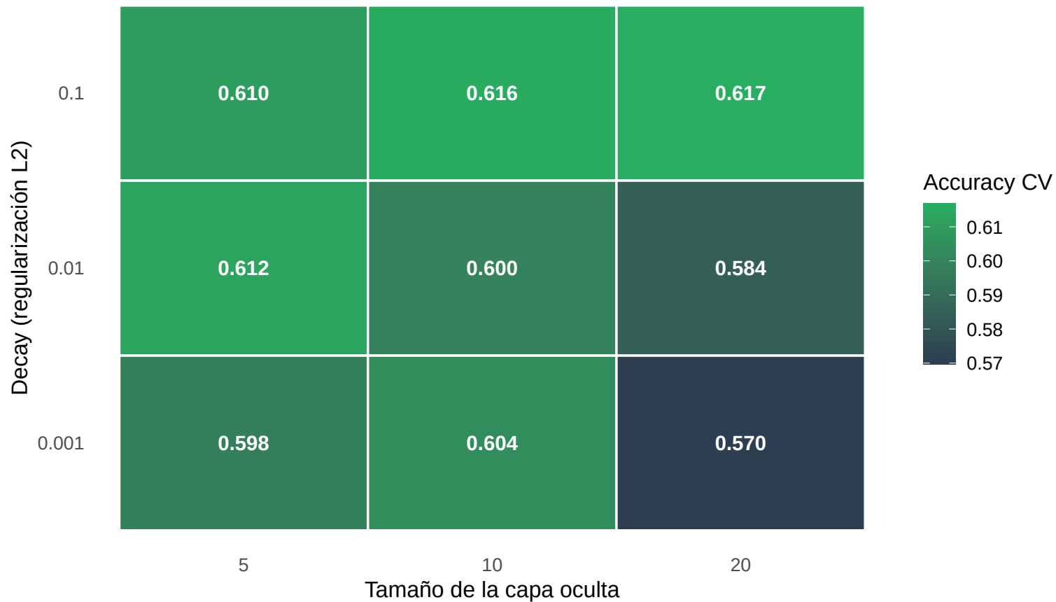
Mapa de calor del barrido de hiperparámetros
