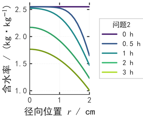
(b) 含水率剖面
