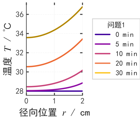
(a) 温度剖面
