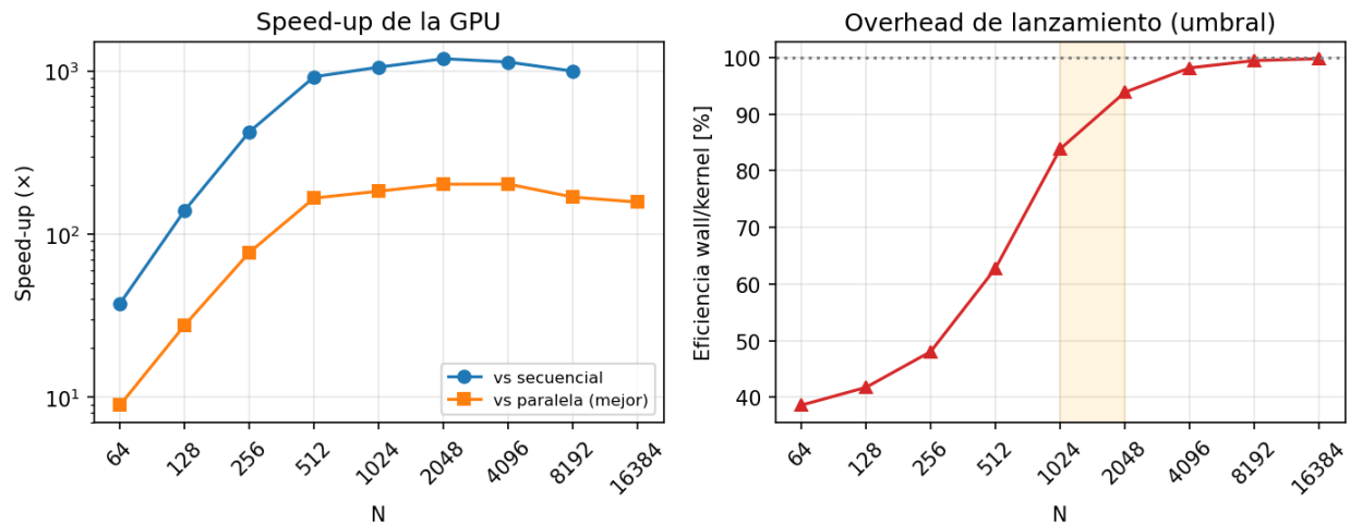
Figura 5: Izquierda: speed-up de la GPU frente a la CPU secuencial y a la mejor paralela. Derecha: eficiencia wall/kernel (peso del overhead de lanzamiento); la banda señala la rodilla N \approx 1024 – 2048 .
