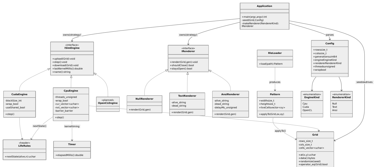
Figura 1: Diagrama de clases del proyecto. La Application posee un ISimEngine y un IRenderer (las dos estrategias). CpuEngine y CudaEngine realizan ISimEngine ; OpenCL está planificado. Las flechas punteadas son dependencias: CpuEngine y CudaEngine usan ambos LifeRules::nextState .
