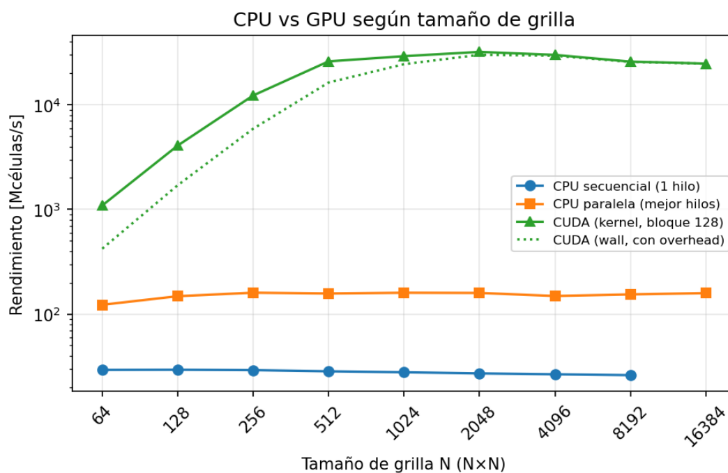
Figura 2: Rendimiento (Mcélulas/s, ejes log-log) según el tamaño de grilla N , mejor de las repeticiones.
