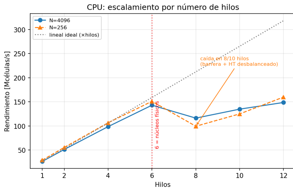
Figura 3: Rendimiento de la CPU (Mcélulas/s) según el número de hilos; la recta punteada es el escalamiento lineal ideal.
