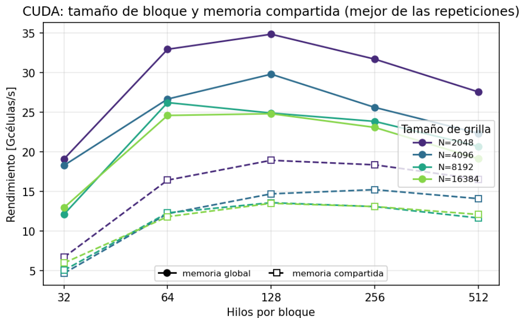
Figura 4: CUDA: rendimiento (Gcélulas/s) por tamaño de bloque, memoria global (sólido) frente a compartida (discontinuo), para varias grillas.
