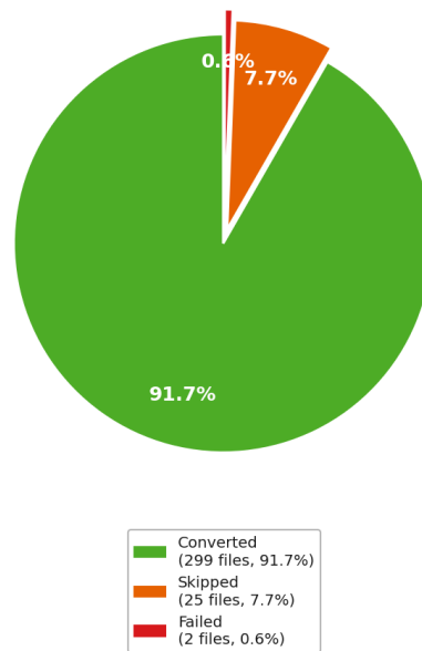
Proporsi Hasil Konversi Rector (CBT DTI -- Qwen2.5-Coder:7b (cibt_qwen) -- Target PHP 8.3)
