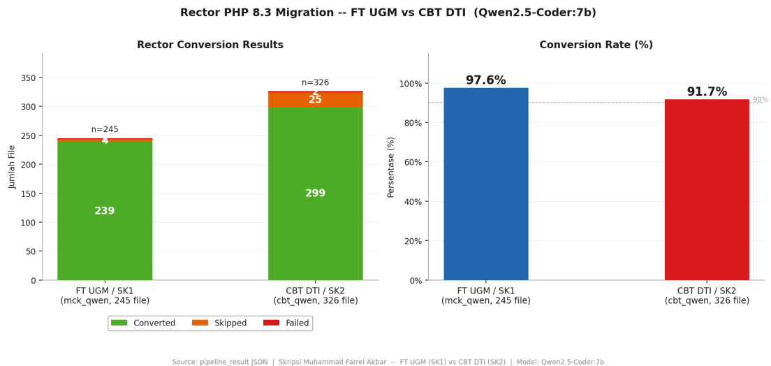
Gambar 4.24. Perbandingan hasil konversi Rector pada kedua studi kasus
