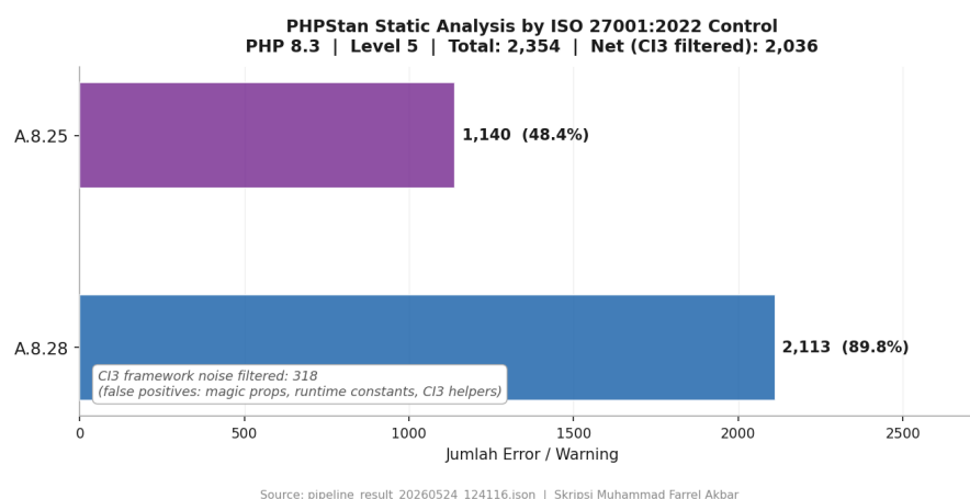
Gambar 4.22. Distribusi temuan PHPStan berdasarkan kontrol ISO/IEC 27001:2022 Annex A pada dataset CBT DTI UGM
