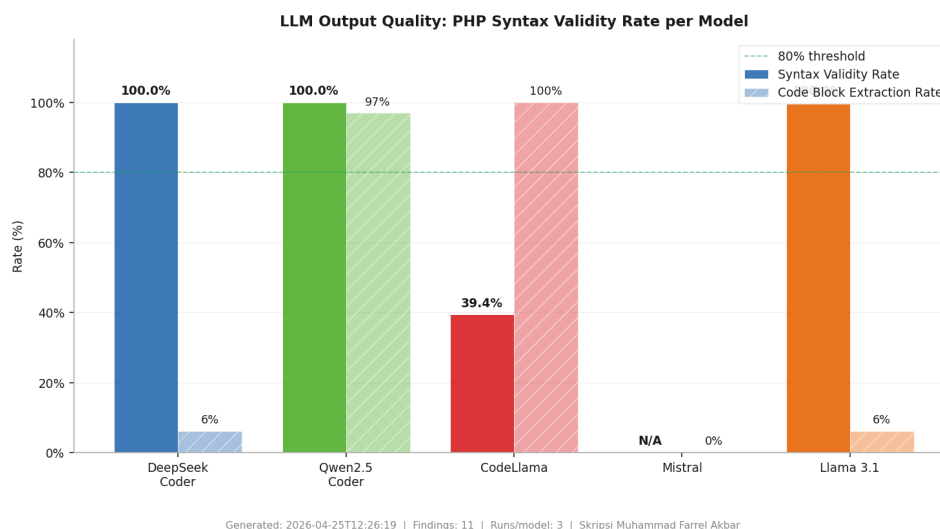
Gambar 4.8. Syntax validity rate dan code block extraction rate kelima model LLM pada Kondisi A
