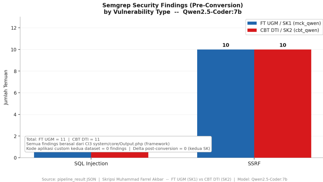
Gambar 4.23. Perbandingan temuan Semgrep pre-scan berdasarkan jenis kerentanan pada kedua studi kasus
