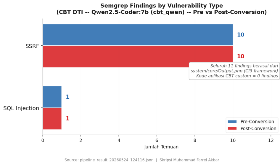
Gambar 4.21. Temuan Semgrep pre-scan vs post-scan berdasarkan jenis kerentanan pada dataset CBT DTI UGM
