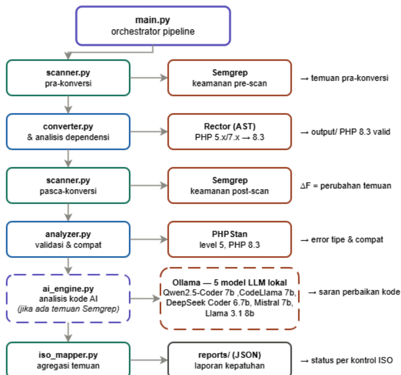
Gambar 3.2. Arsitektur sistem pipeline dengan enam modul fungsional dan satu orkestrator
