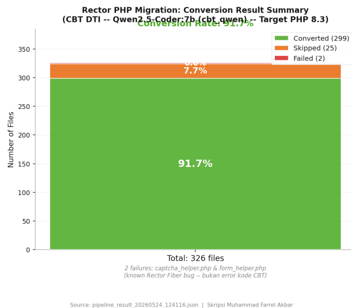
Gambar 4.18. Ringkasan hasil konversi Rector terhadap 326 file PHP dataset CBT DTI UGM (diagram batang)
