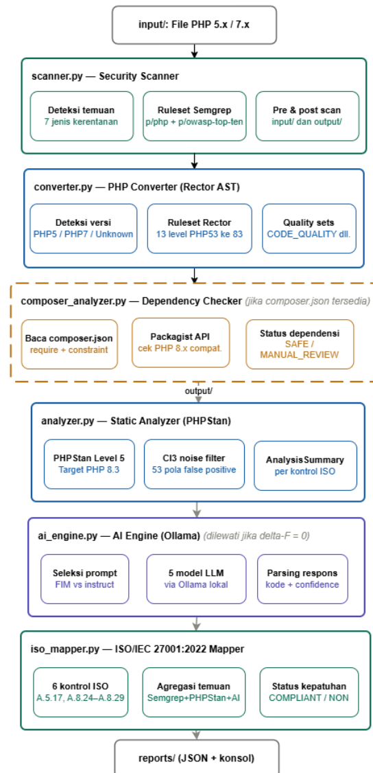
Gambar 3.3. Alur data pipeline dari input hingga laporan akhir
