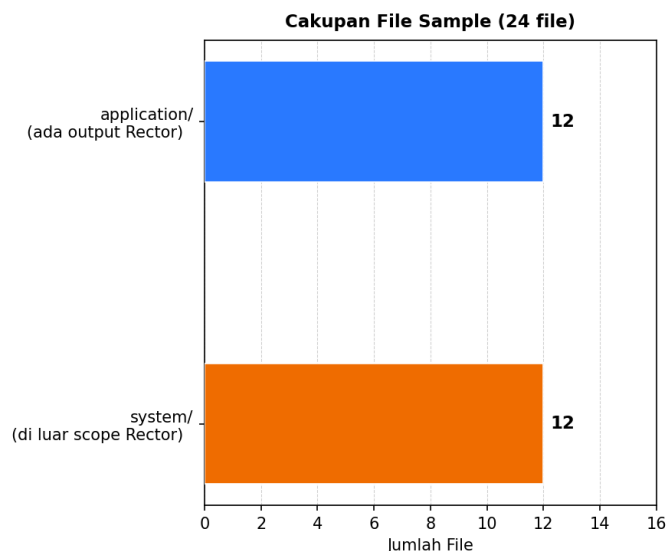
Gambar 4.13. Distribusi cakupan file sampel validasi 24 file berdasarkan direktori asal
