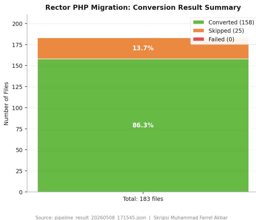
Gambar 4.13. Ringkasan hasil konversi Rector terhadap 183 file PHP dataset CBT DTI UGM
