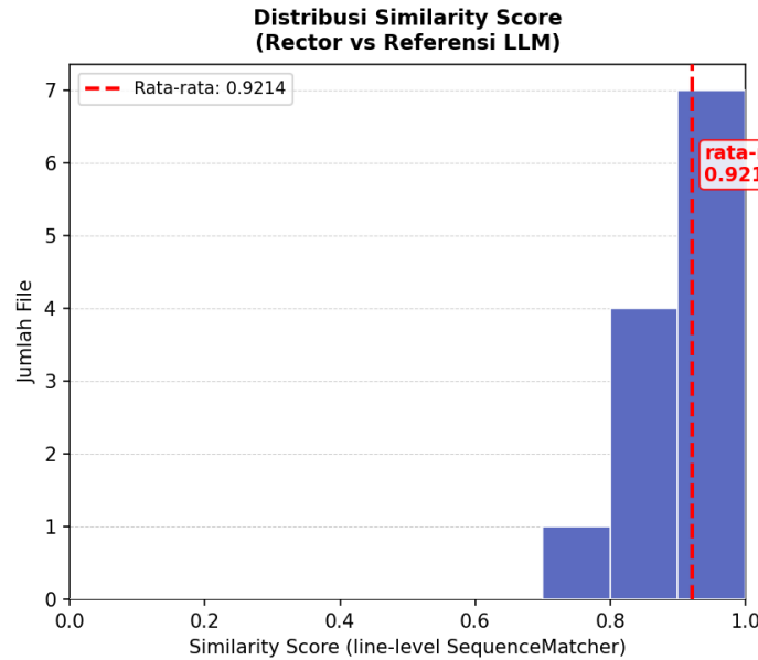
Gambar 4.15. Distribusi similarity score antara keluaran Rector dan referensi LLM pada 12 file sampel ( line-level SequenceMatcher )
