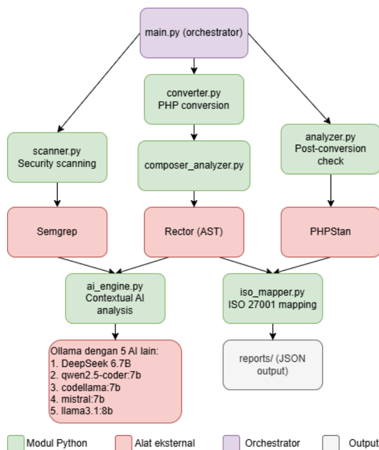
Gambar 3.2. Arsitektur sistem pipeline dengan enam modul fungsional dan satu orkestrator
