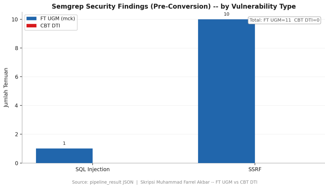
Gambar 4.23. Perbandingan temuan Semgrep pre-scan berdasarkan jenis kerentanan pada kedua studi kasus
