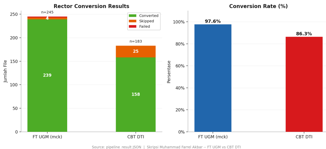
Gambar 4.24. Perbandingan hasil konversi Rector pada kedua studi kasus
