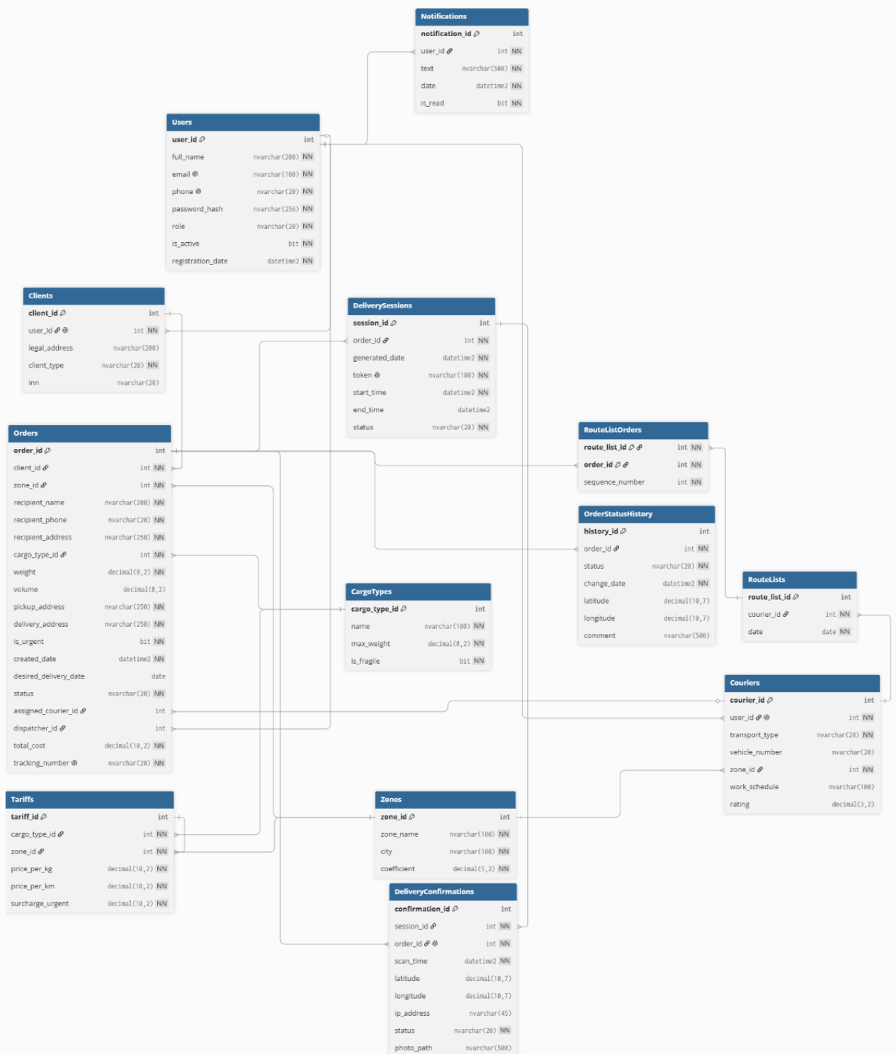
Рисунок 3 — ER-диаграмма базы данных системы «FastDelivery»
