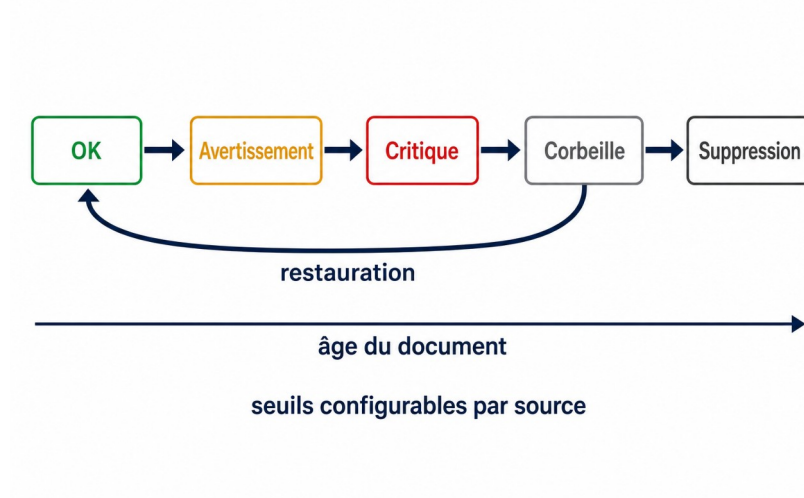
Figure 4 : Cycle de vie d'un document PDF : états de fraîcheur, transitions et chronologie de purge.
