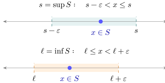
Figura 1.8. Aproximación al supremo y al ínfimo. Cada franja contiene al menos un elemento de S para todo \varepsilon > 0 ; no se afirma que la franja entera pertenezca a S .
