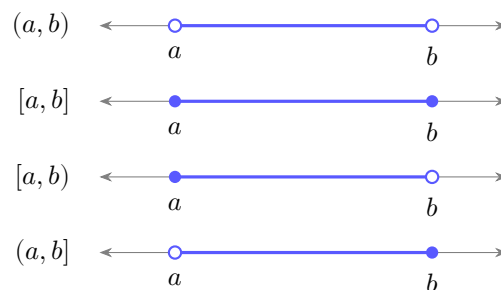
Figura 1.3. Intervalos acotados y pertenencia de sus extremos.
