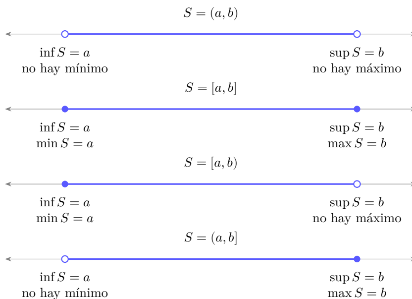
Figura 1.10. Los cuatro intervalos tienen ínfimo a y supremo b . Un punto relleno indica que el extremo pertenece al conjunto y es, además, mínimo o máximo; un punto hueco indica que no se alcanza.
