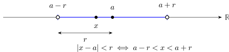
Figura 1.5. El valor absoluto como distancia a un centro.
