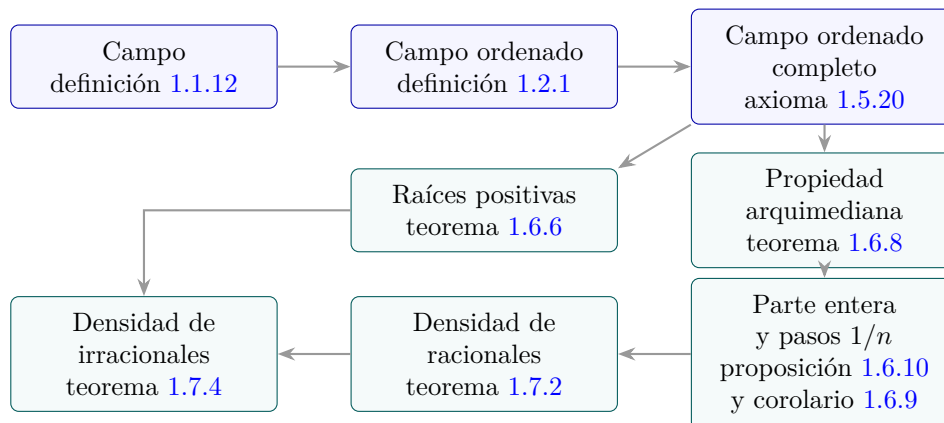
Figura 1.13. Estructuras y resultados del capítulo. Las primeras flechas añaden propiedades a un campo; las restantes indican herramientas utilizadas en las demostraciones. La construcción de irracionales también utiliza la irracionalidad de \sqrt{2} de la proposición 1.1.10.
