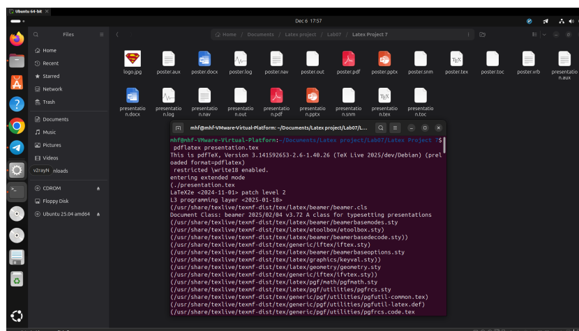
Рис. 9: Компиляция презентации
