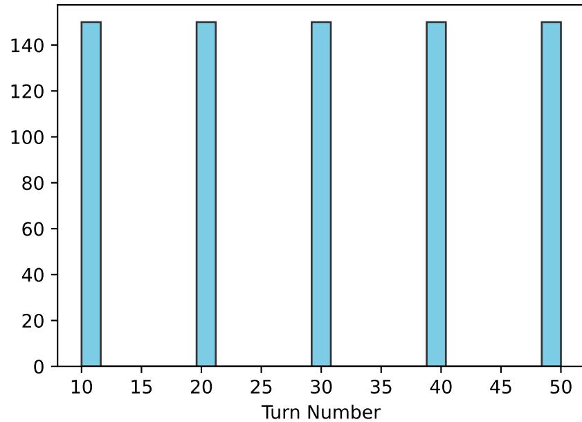
FixedSchedule
