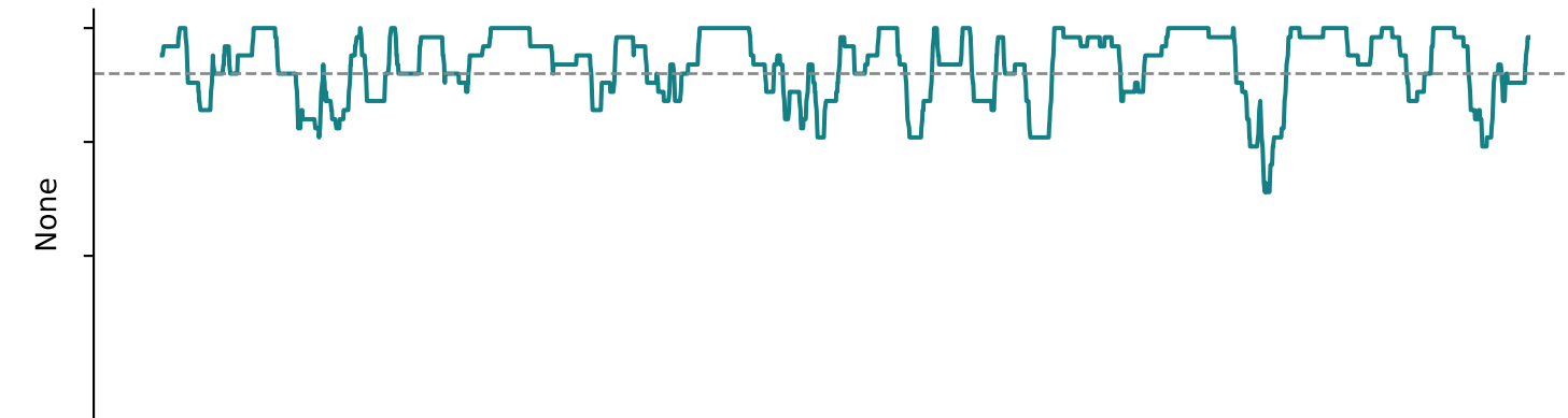
Ours
