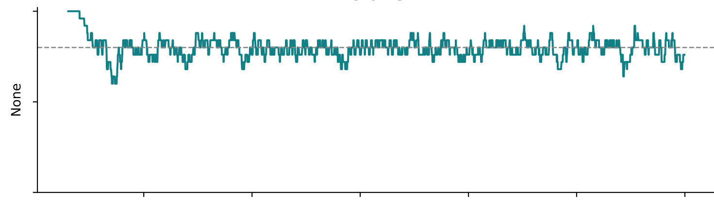
Ours
