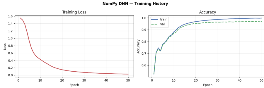
Fig. 1. Resultados do treino do modelo NumPy DNN.
