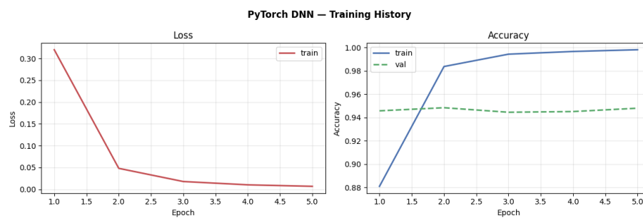
Fig. 2. Resultados do treino do modelo PyTorch DNN.
