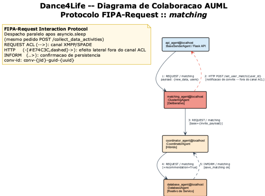
Fig. 7. Diagrama de colaboração AUML Protocolo FIPA-Request, ontologia matching . A mensagem 2 representa o efeito lateral HTTP (POST /set_user_match/{id}) que o ClusteringAgent efectua directamente sobre a Flask API fora do canal ACL , antes de encaminhar o resultado via XMPP para o CoordinatorAgent (mensagem 3).
