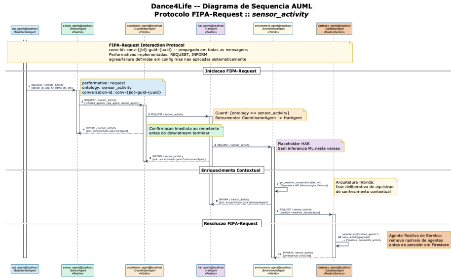
Fig.8. Diagrama de sequência AUML Protocolo FIPA-Request, ontologia sensor_activity . 11 mensagens numeradas: REQUEST 1–3, 5, 9 (setas sólidas); INFORM 4, 6, 8, 11 (setas tracejadas); auto-mensagens 7 ( get_weather_temperature ) e 10 ( save_activity ). Os blocos de ativação mostram o período em que cada agente aguarda resposta do downstream.
