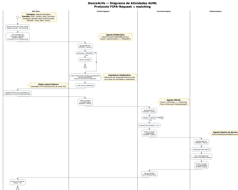
Fig. 4. Diagrama de atividades AUMIL Protocolo FIPA-Request, ontologia matching . Fluxo: API → ClusteringAgent (inferência deliberativa) → notificação HTTP lateral ( /set_user_match ) → CoordinatorAgent → DatabaseAgent. Retorno INFORM de DatabaseAgent para CoordinatorAgent.
