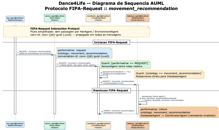
Fig.9. Diagrama de sequência AUML Protocolo FIPA-Request, ontologia movement_recommendation . Fluxo de 6 mensagens: REQUEST 1-2 (APISensorAgentCoordinatorAgent), auto-mensagem 3 ( payload["recommendation"]=True ), REQUEST 4 (DatabaseAgent), auto-mensagem 5 ( save_movement_recommendation ) e INFORM 6 de confirmação.
