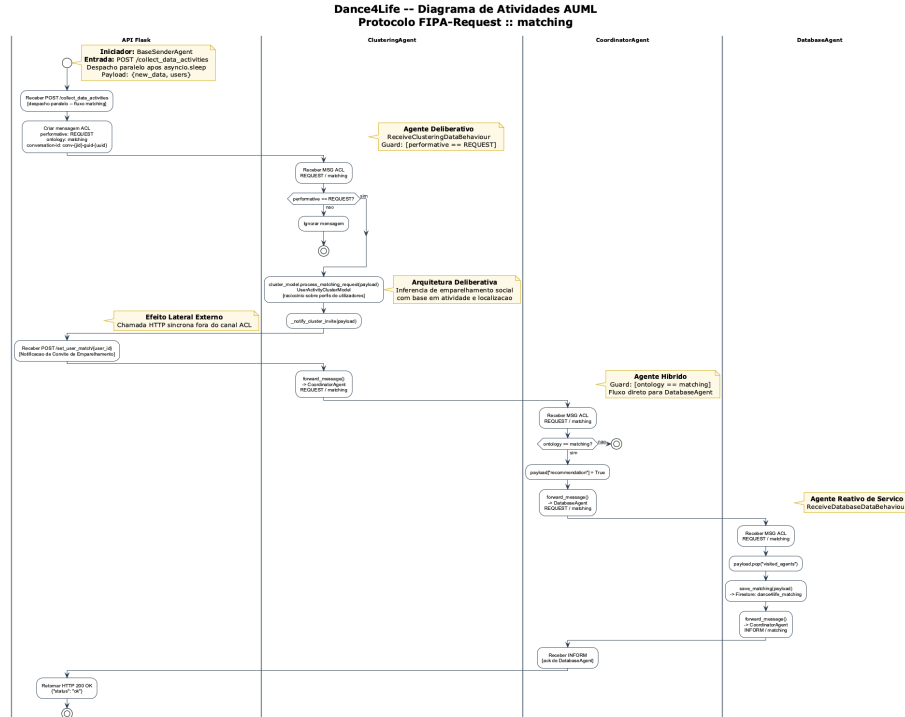
Fig. 4. Diagrama de actividades AUML Protocolo FIPA-Request, ontologia matching . Fluxo: API → ClusteringAgent (inferência deliberativa) → notificação HTTP lateral ( /set_user_match ) → CoordinatorAgent → DatabaseAgent. Retorno INFORM de DatabaseAgent para CoordinatorAgent.
