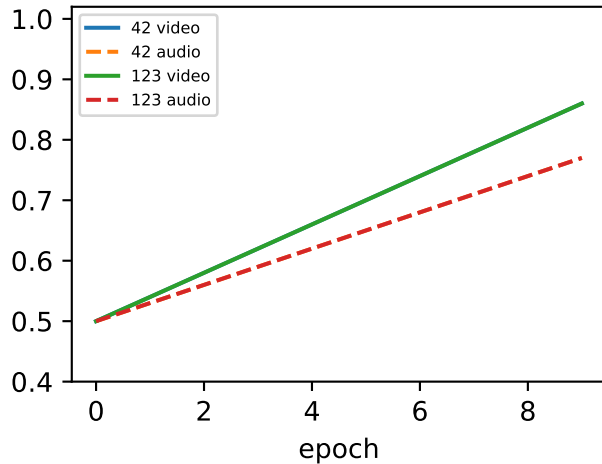
Validation AUC
