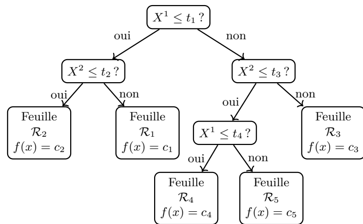
Arbre de décision correspondant (règles si-alors)
