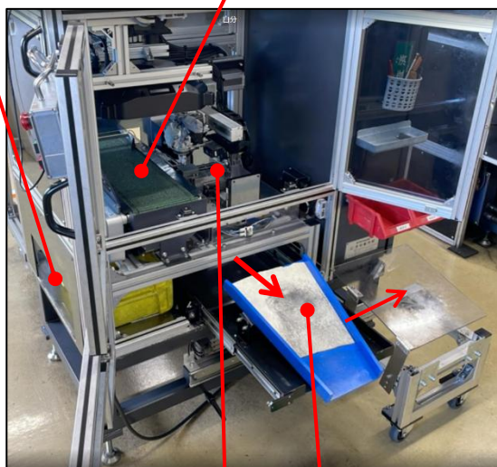
機械正面
