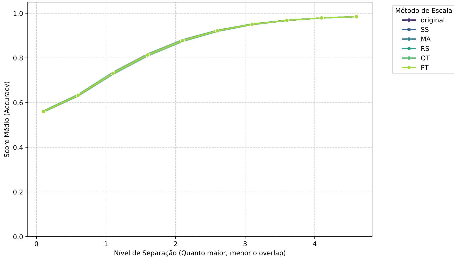
Média Geral: AdaBoost - ACCURACY vs Separação
