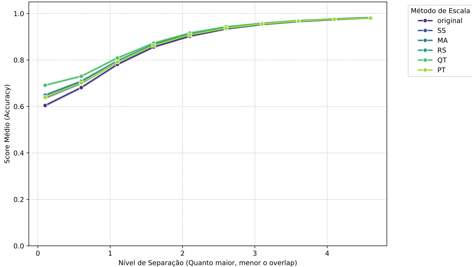
Média Geral: KNORAU - ACCURACY vs Separação
