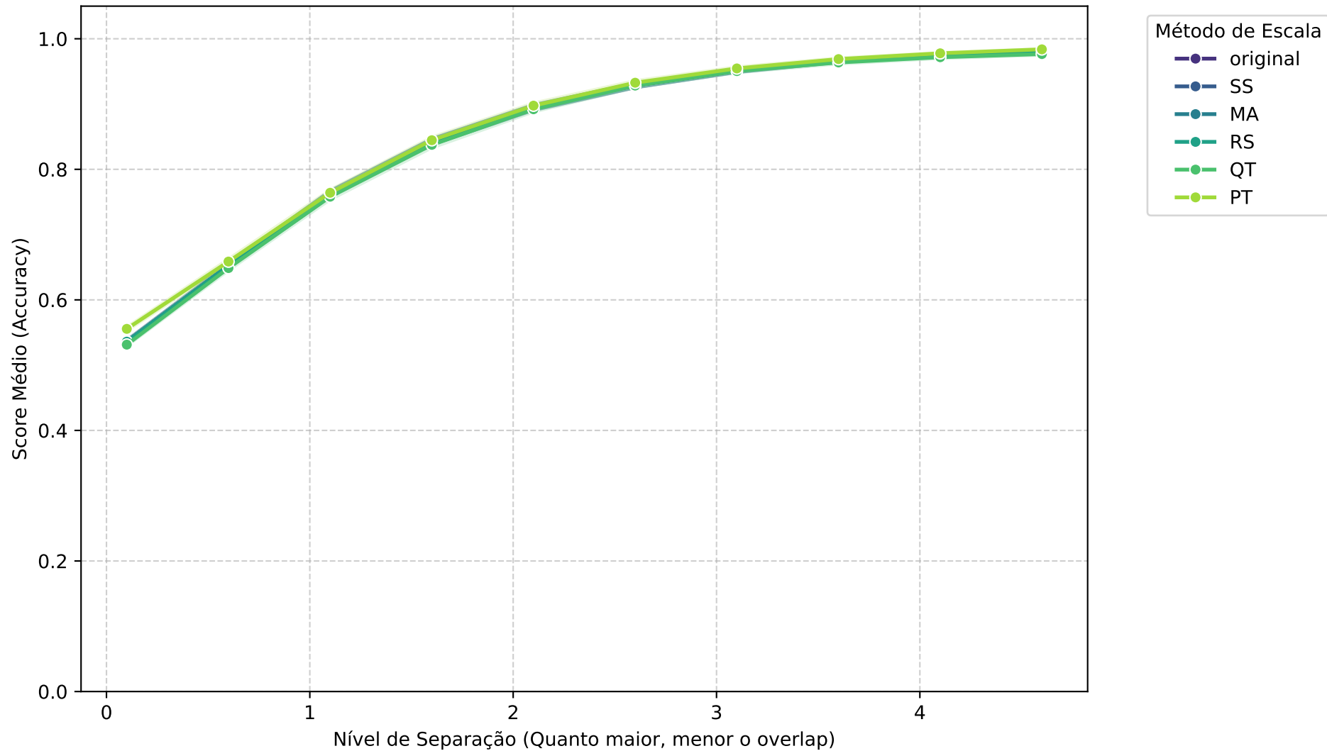
Média Geral: LDA - ACCURACY vs Separação
