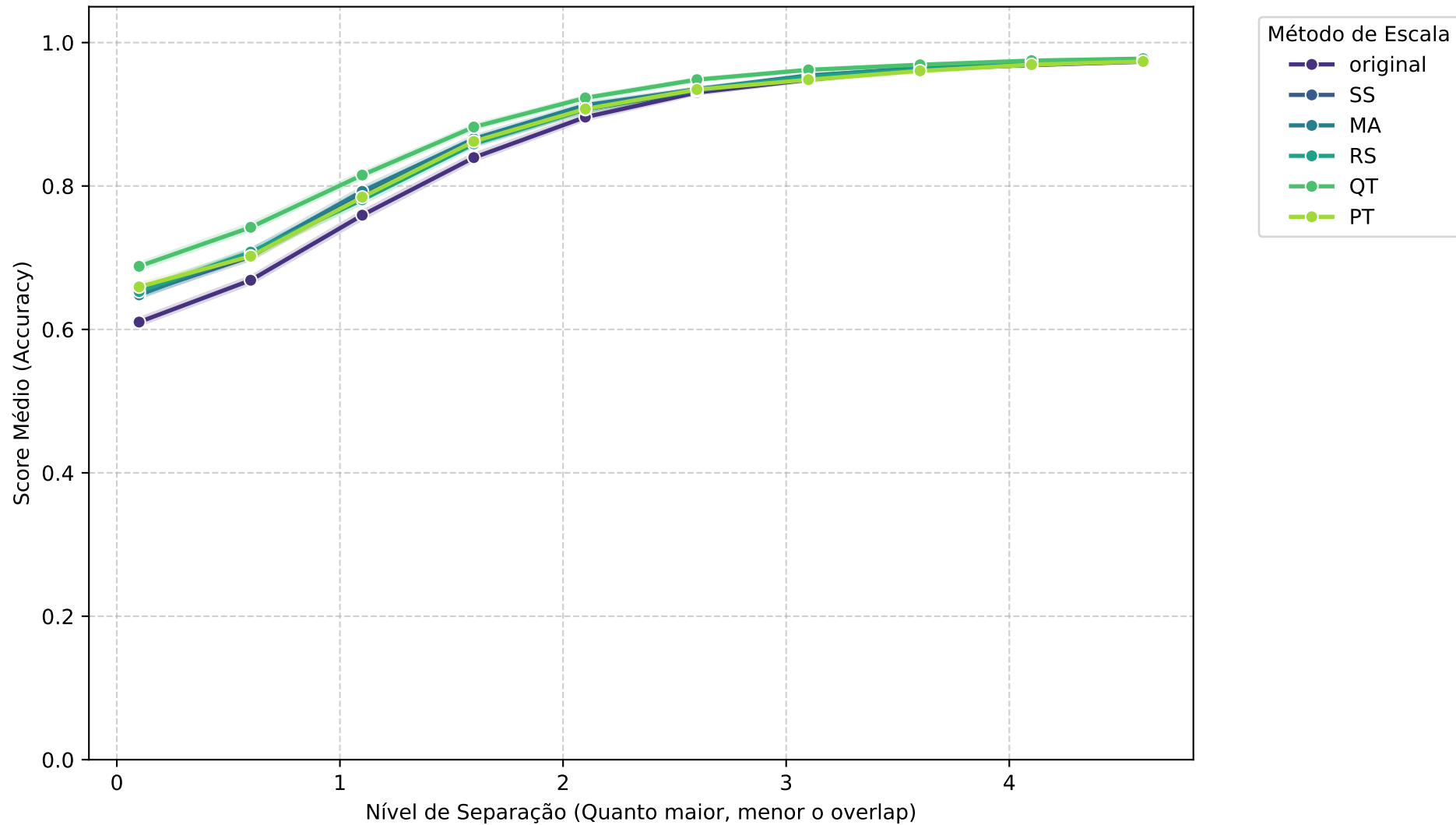
Média Geral: MCB - ACCURACY vs Separação
