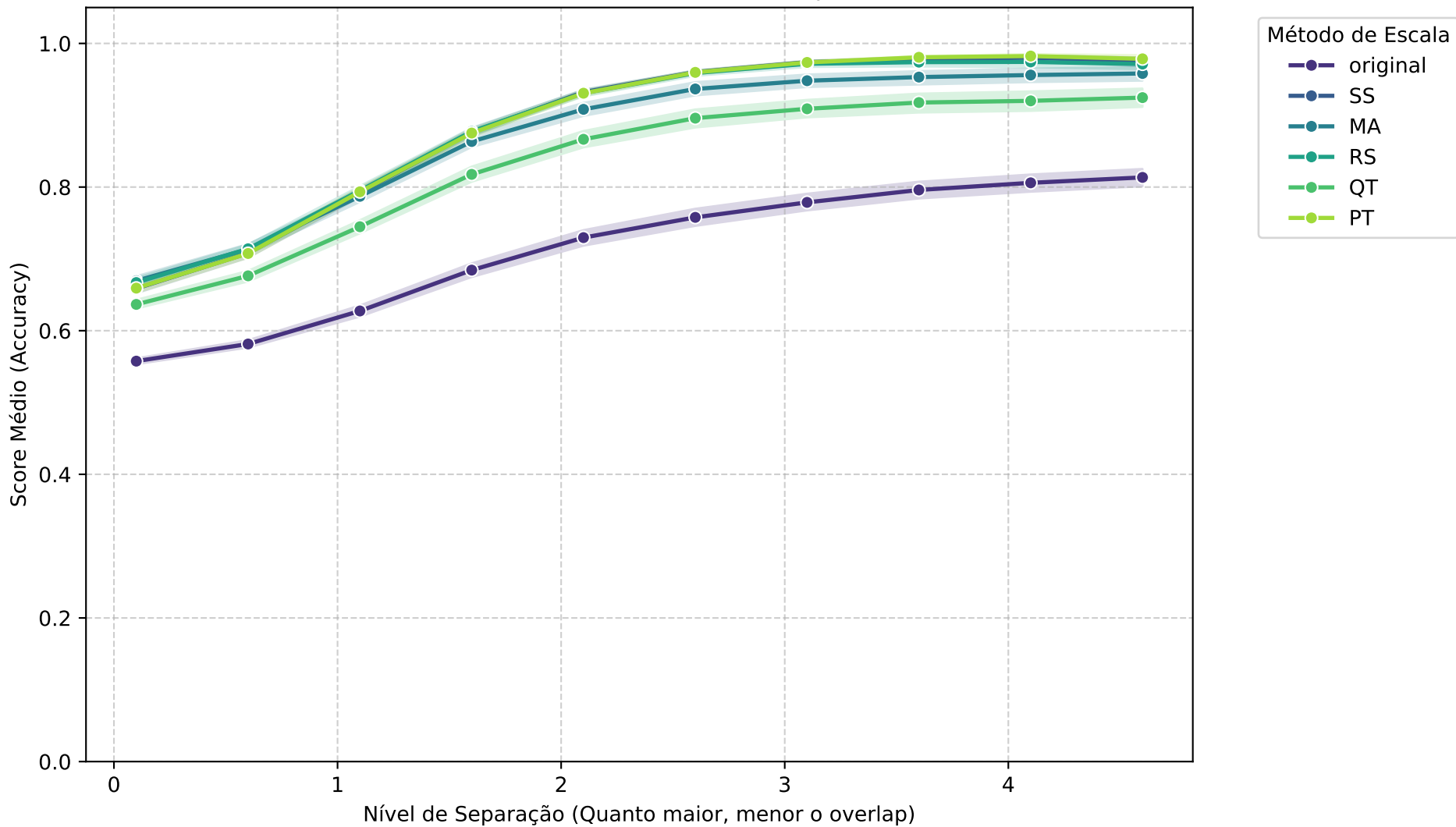
Média Geral: MLP - ACCURACY vs Separação
