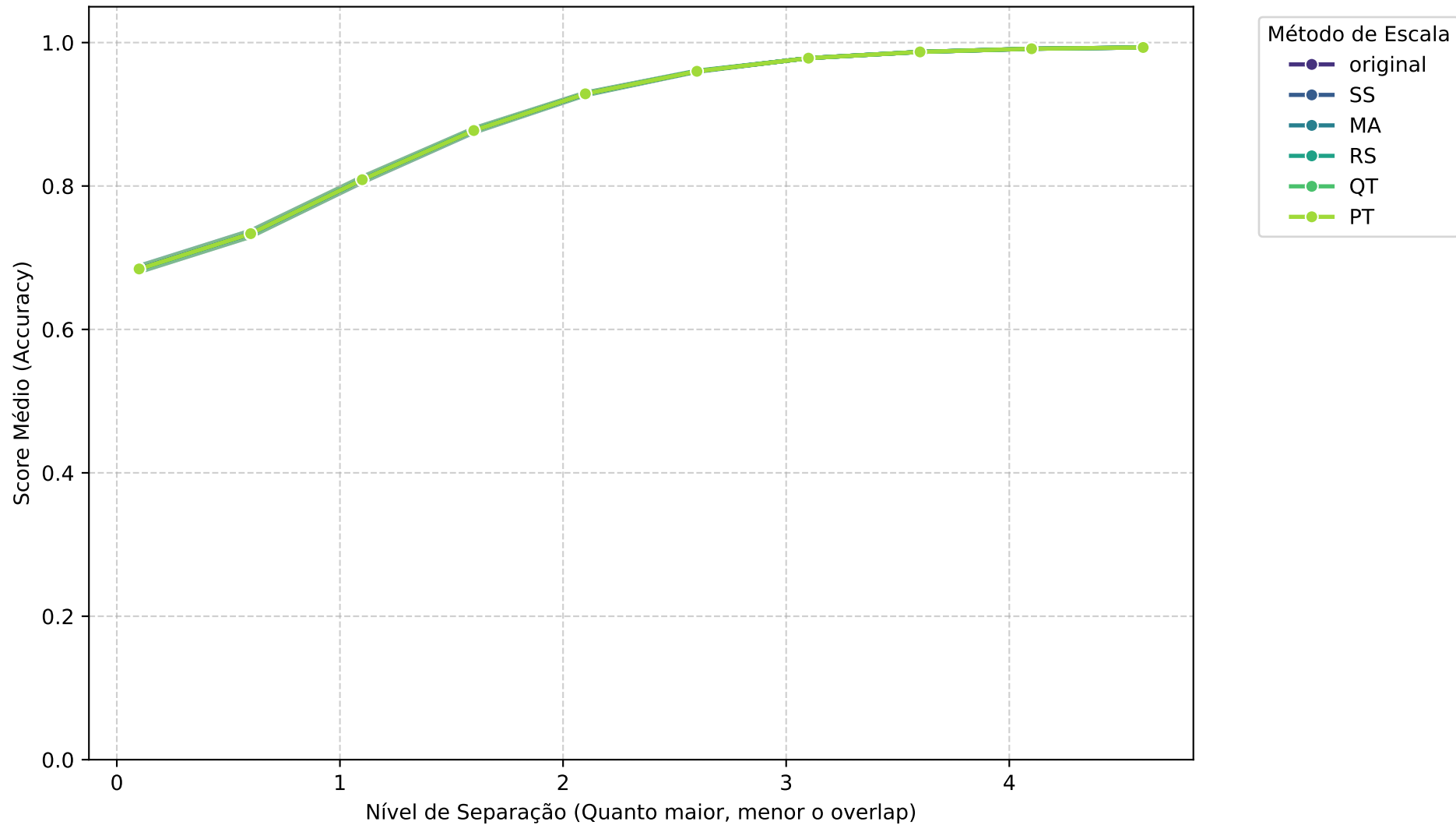
Média Geral: RF - ACCURACY vs Separação
