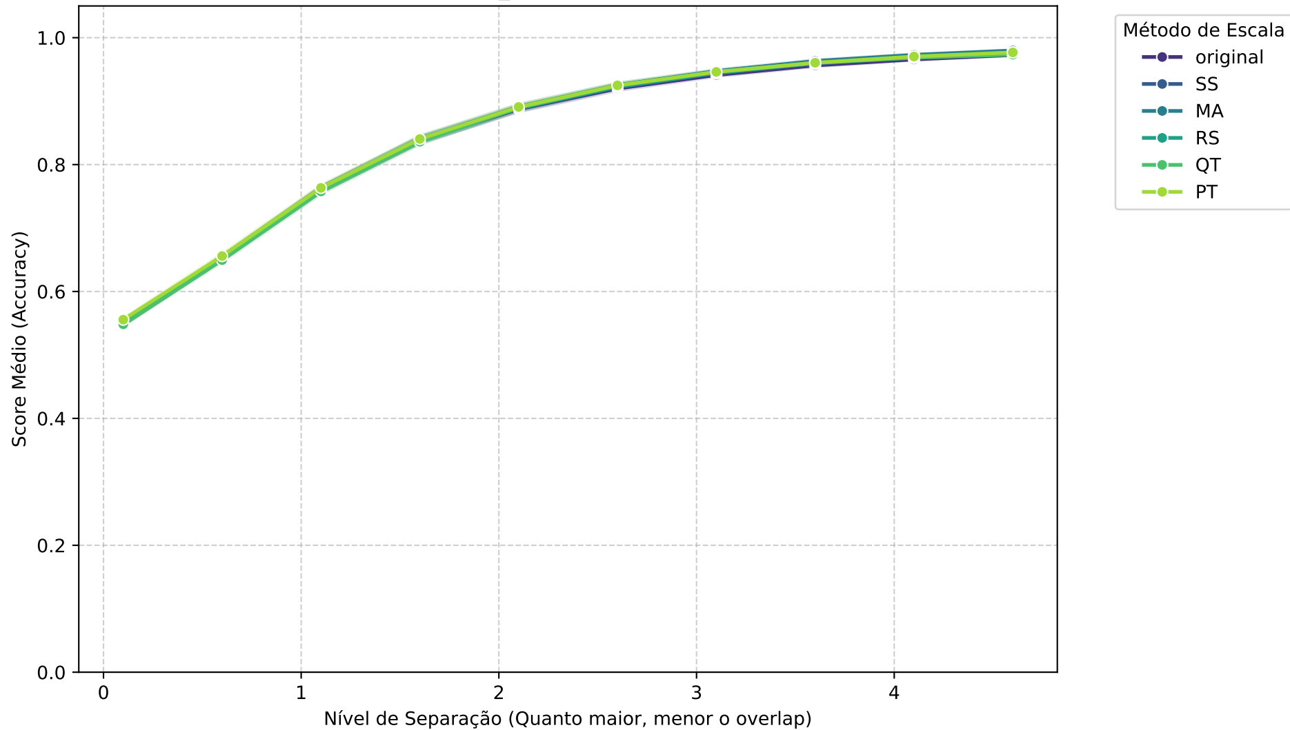
Média Geral: SVM_lin - ACCURACY vs Separação
