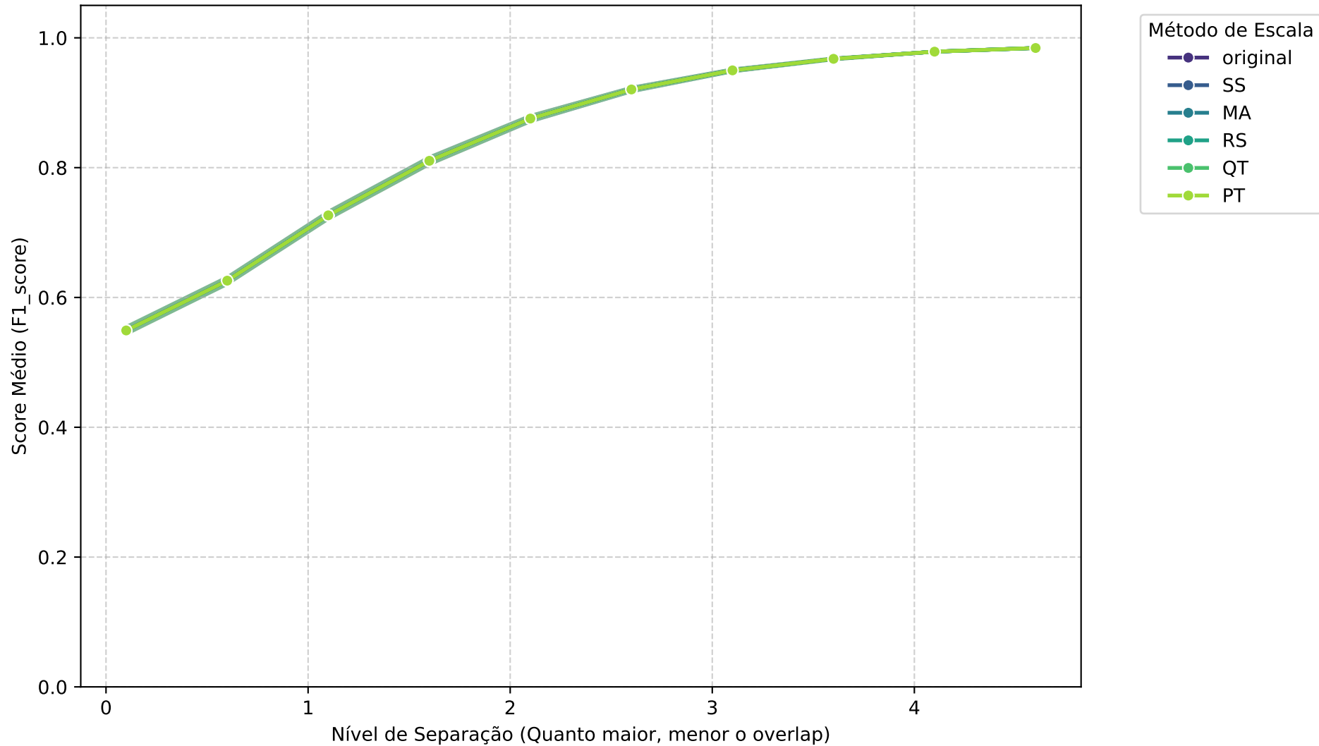
Média Geral: AdaBoost - F1_SCORE vs Separação
