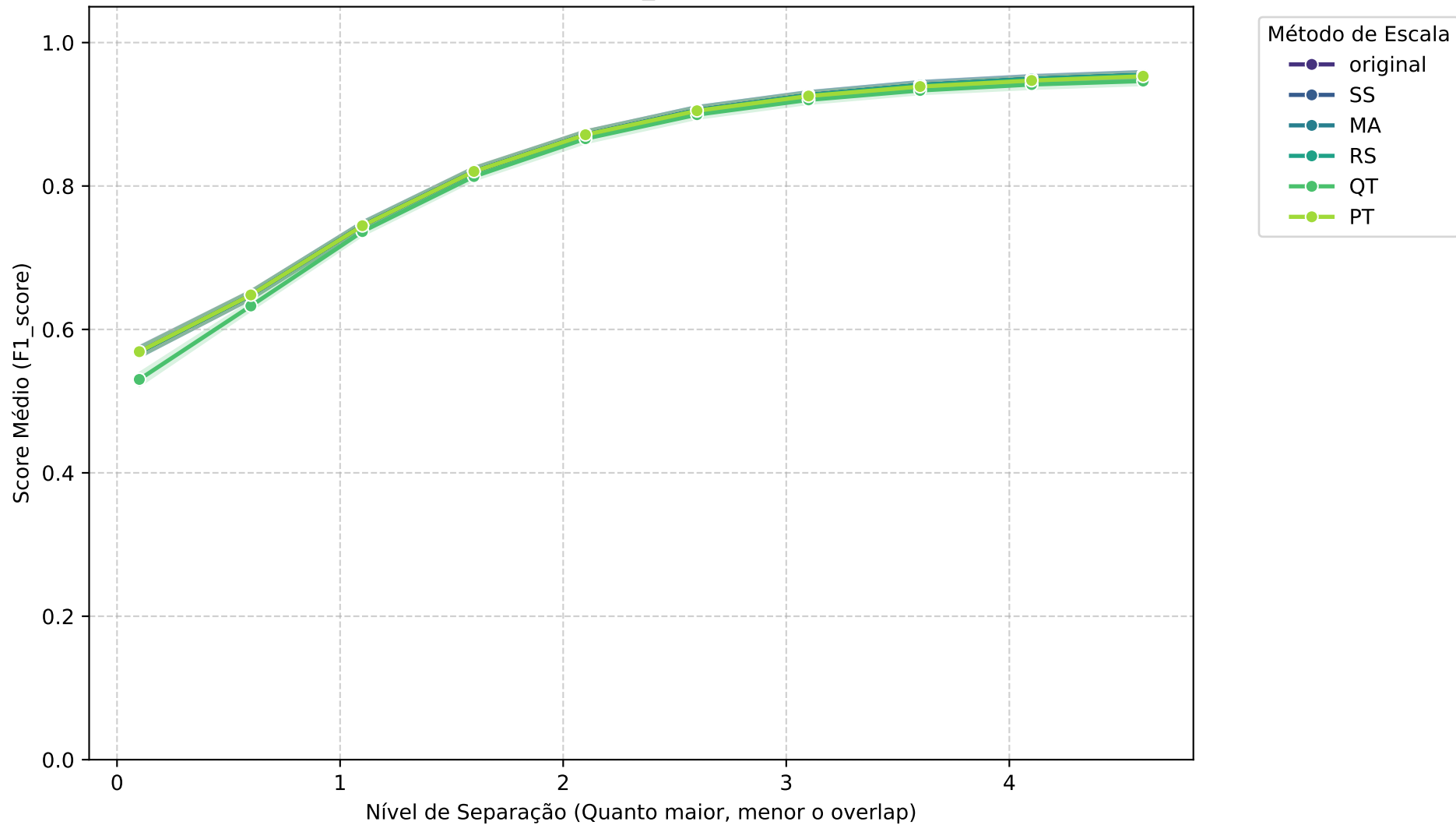
Média Geral: GNB - F1_SCORE vs Separação
