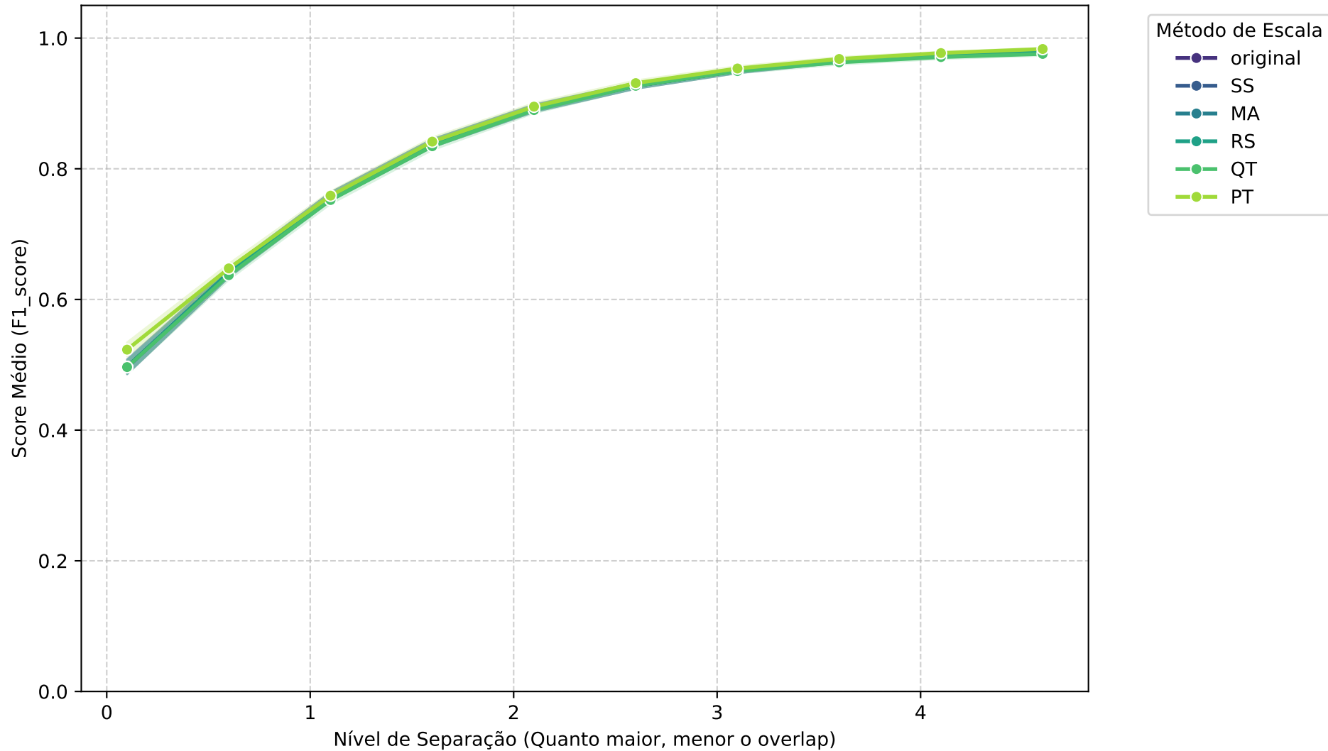
Média Geral: LDA - F1_SCORE vs Separação
