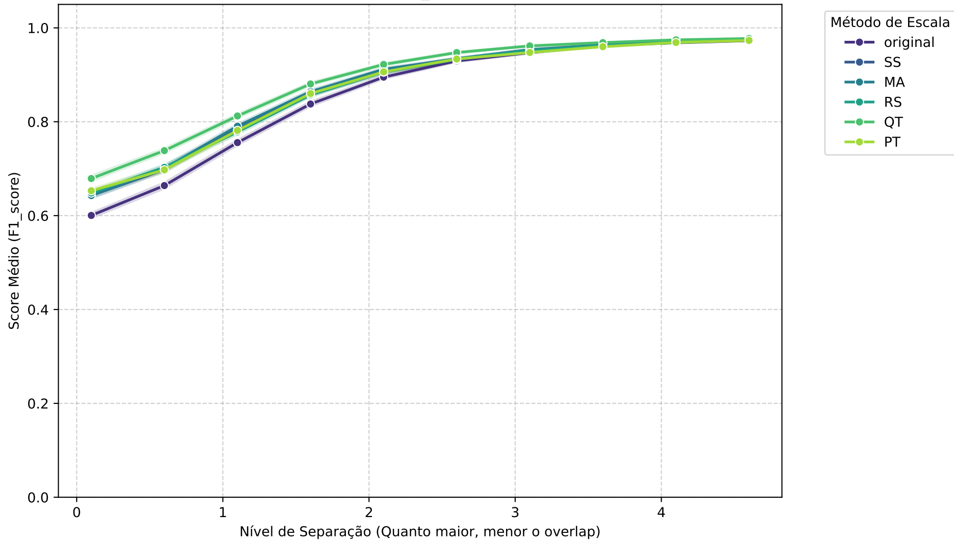
Média Geral: MCB - F1_SCORE vs Separação
